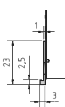
typ 3 mm
